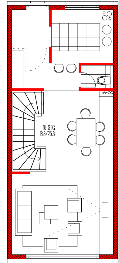
MITTELHAUSBEISPIEL (1:100)
