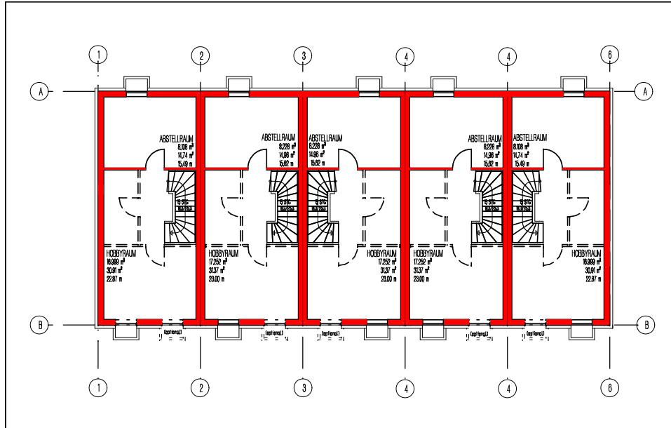
ÜBERSICHT UG (1:250)
